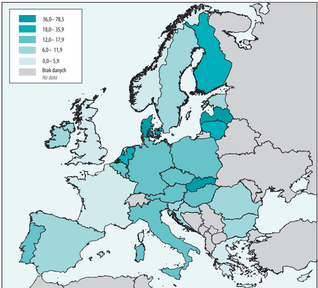
Udział kogeneracji w produkcji energii elektrycznej w 2016 r. (%) Share of combined heat and power (CHP) in gross electricity generation in 2016 (%)
